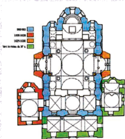
Plan du catholicon du monastère d'Iviron
